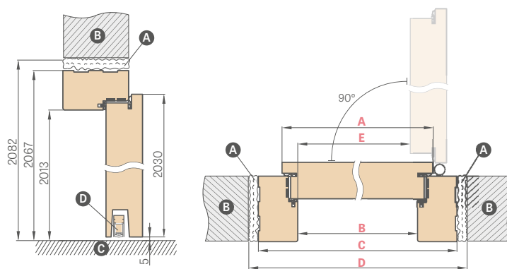
PRZEKRÓJ OŚCIEŻNICY P.POŻ Z PODSTAWOWĄ ZABUDOWĄ MURU
