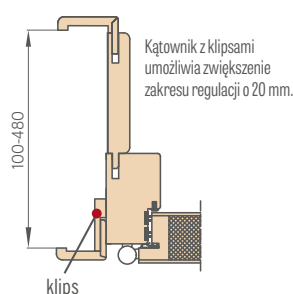
PRZEKRÓJ OŚCIEŻNICY P.POŻ Z ZABUDOWĄ MURU I KĄTOWNIKIEM Z KLIPSEM
