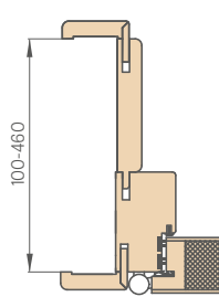
PRZEKRÓJ OŚCIEŻNICY P.POŻ Z PODSTAWOWĄ ZABUDOWĄ MURU
