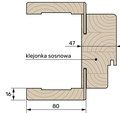
Panel pojedynczy
